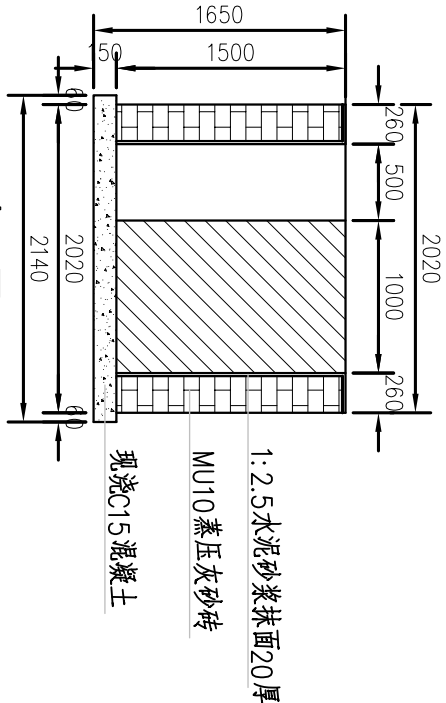
B-B断面图 1:50
