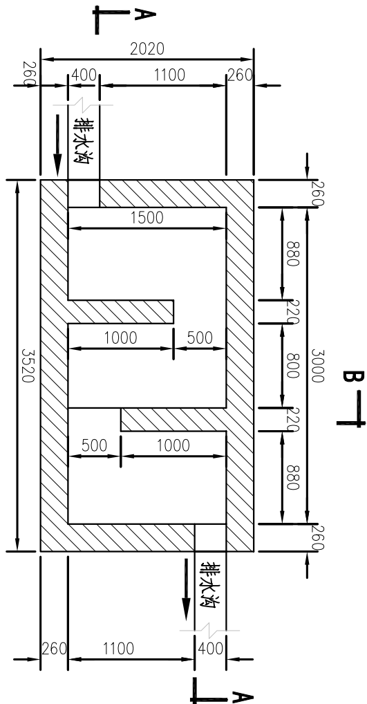
沉沙池平面图 (主体设计/方案新增) 1:50
