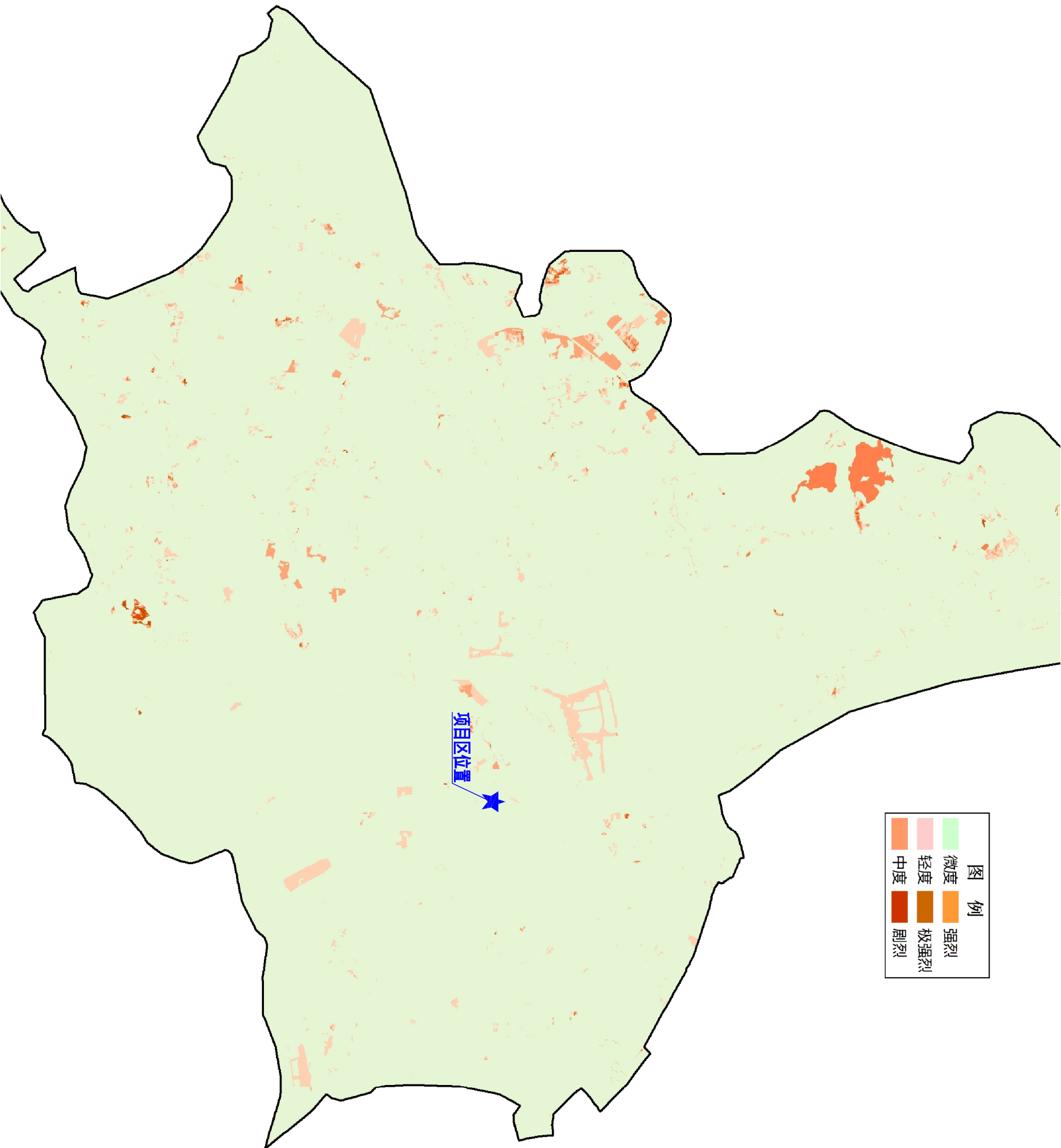
项目区土壤侵蚀强度分布图
