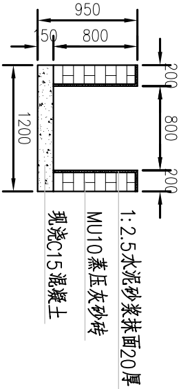
集水井大样图 (主体设计) 1:50
