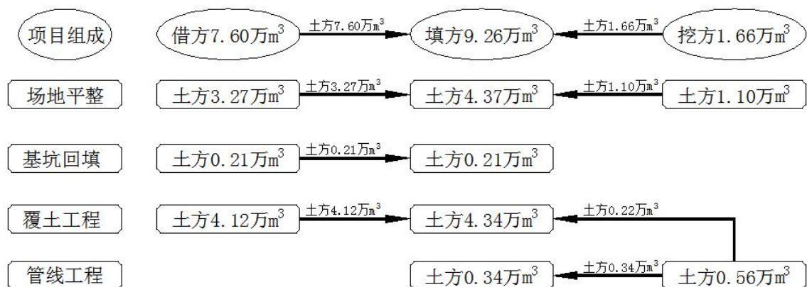
图 2.4-1 土石方流向框图
