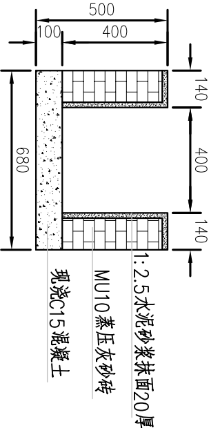
基坑排水沟大样图 (主体设计) 1:20
